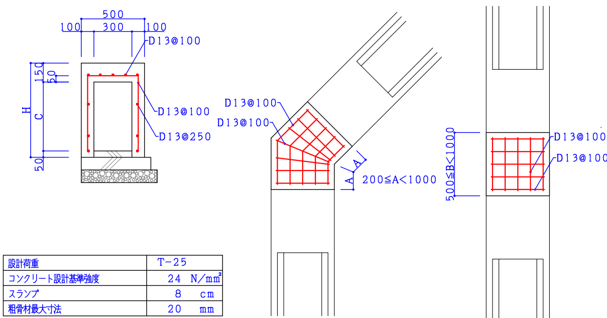
勾配可変側溝端部処理部
