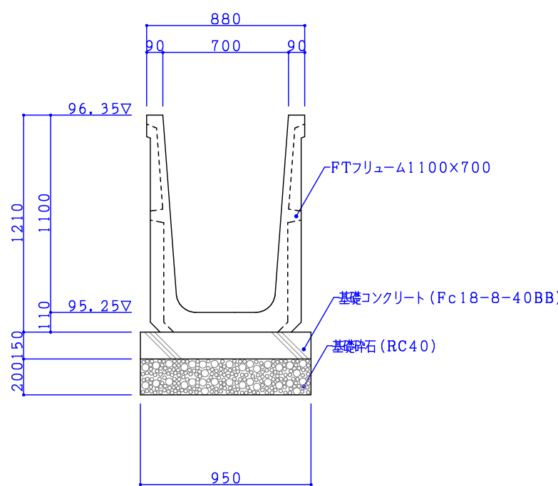
FTフリームΔ1100×700
